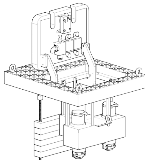
ПИТ-система тип В в открытом положении
