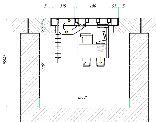
ПИТ-система тип В
