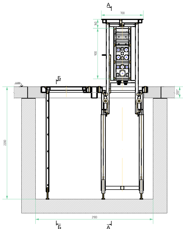
ПИТ-система тип Лифт Стандарт в рабочем положении
