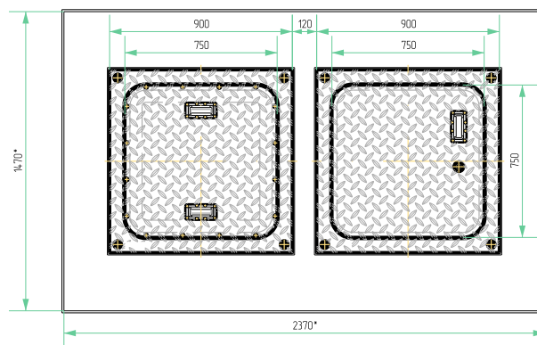
ПИТ-система тип Лифт Соло (рядом зона для обслуживания) вид сверху
