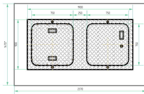
ПИТ-система тип Лифт Стандарт вид сверху
