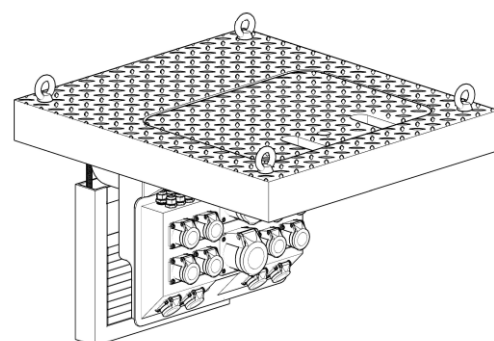
ПИТ-система тип А в закрытом положении
