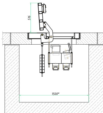
ПИТ-система тип В
