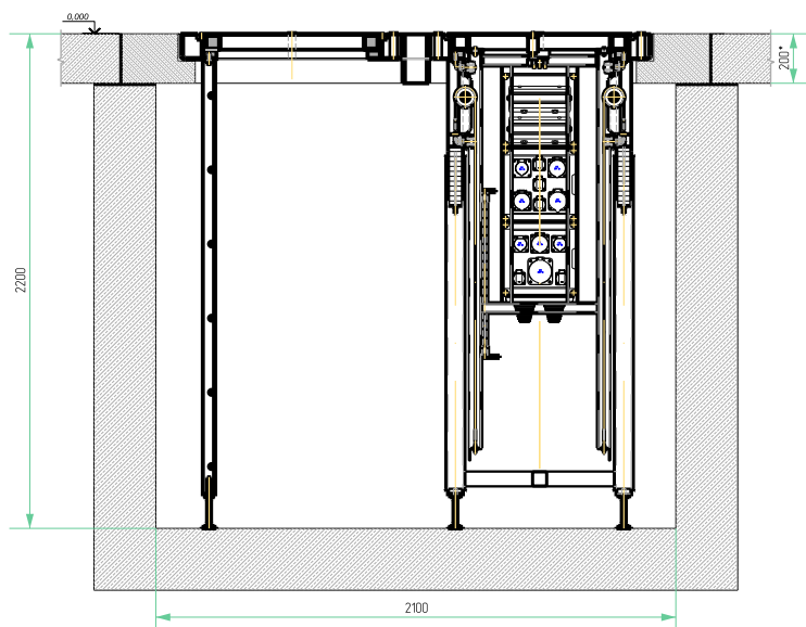
ПИТ-система тип Лифт Стандарт в закрытом положении
