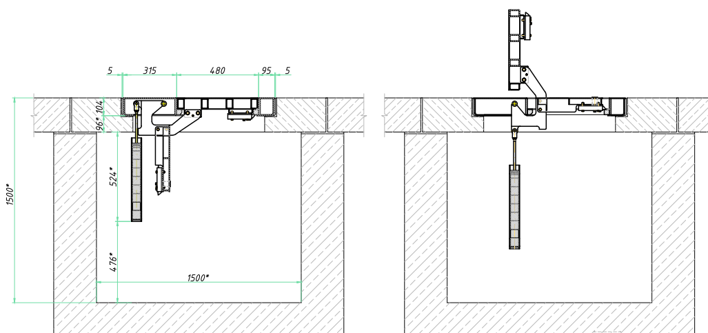
Разрез (ПИТ-система тип А)
