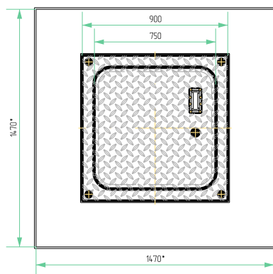
ПИТ-система тип Лифт Соло вид сверху
