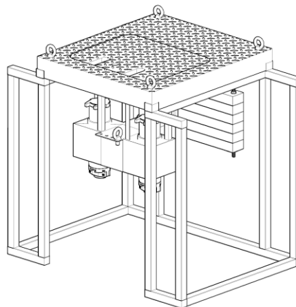
ПИТ-система на станине
