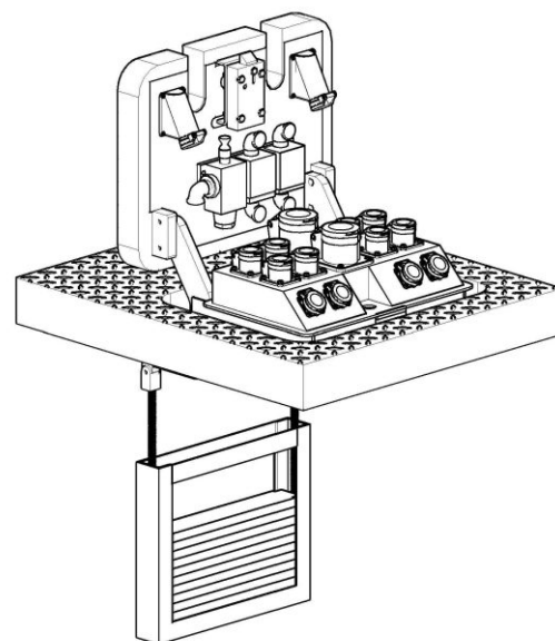
ПИТ-система тип А в открытом положении
