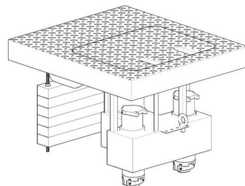
ПИТ-система тип В в закрытом положении
